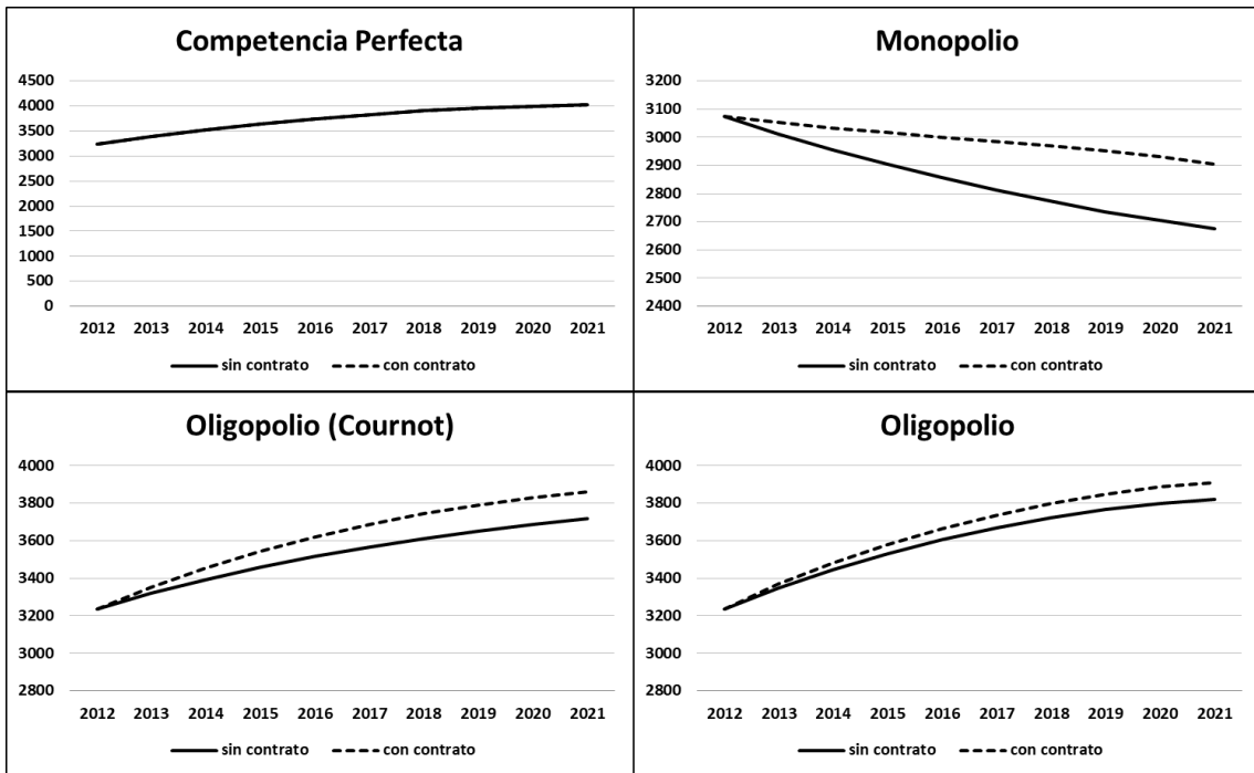
Gráfico 5: Capacidad de generación hidráulica (MW)
