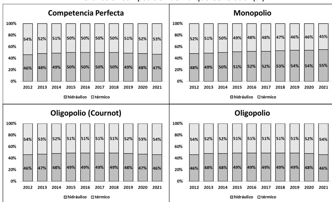
Gráfico 9: Composición del Parque Generador (%)
