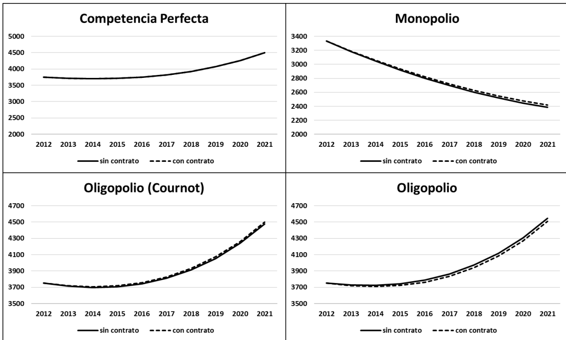
Gráfico 6: Capacidad de generación térmica (MW)
