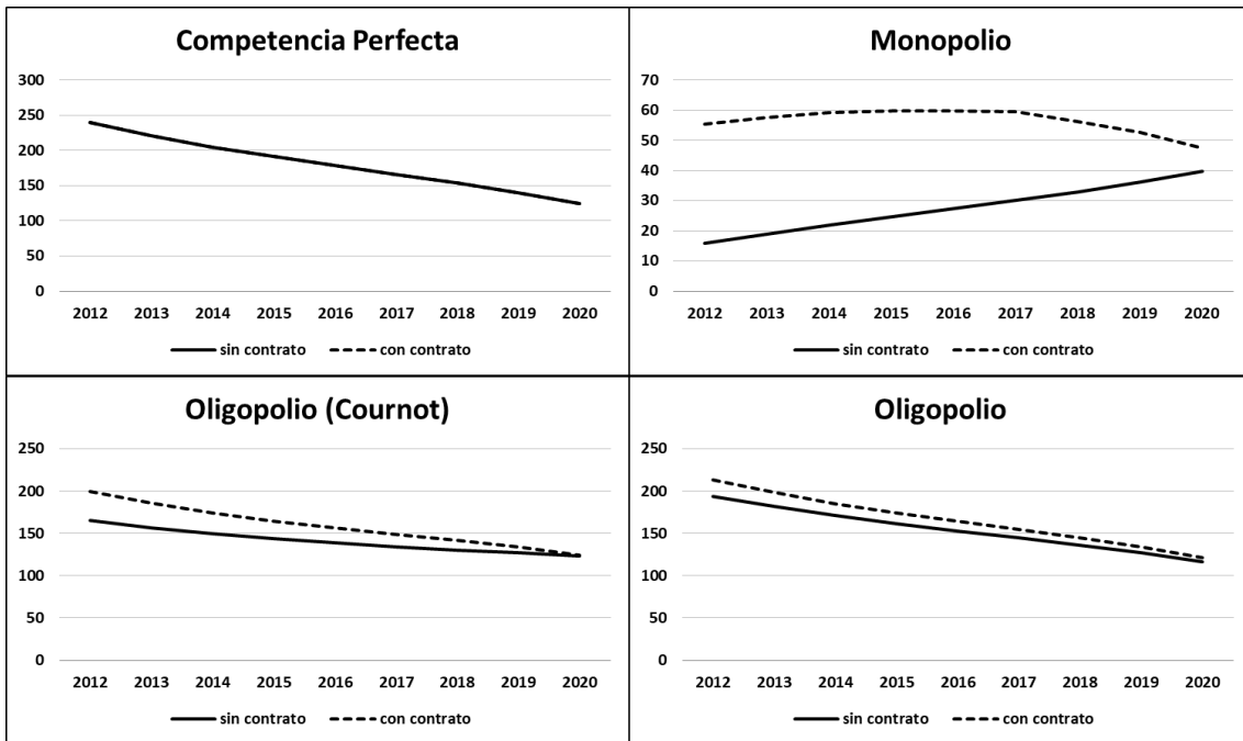
Gráfico 3: Inversión en tecnología hidráulica (MW)
